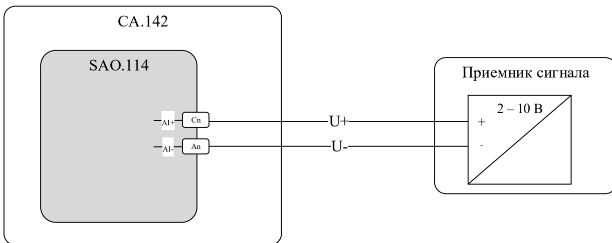
Рисунок В.2 – Схема типового подключения сигналов выдачи напряжения без резервирования блоков
