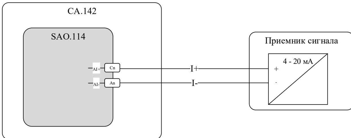
Рисунок В.1 – Схема типового подключения сигналов выдачи постоянного тока без резервирования блоков
